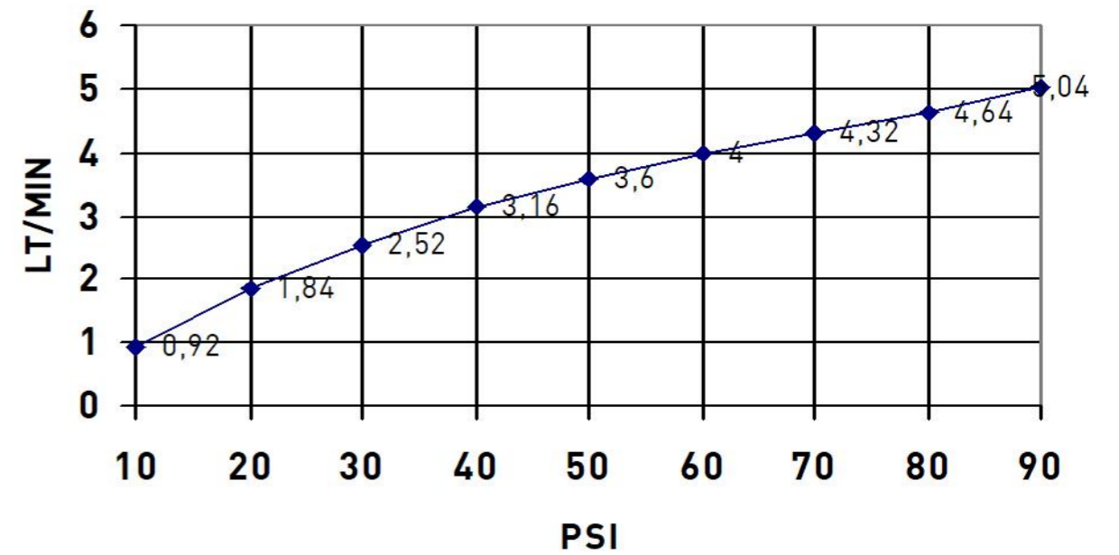
GRAFICO PORTATA / FLOW RATE
